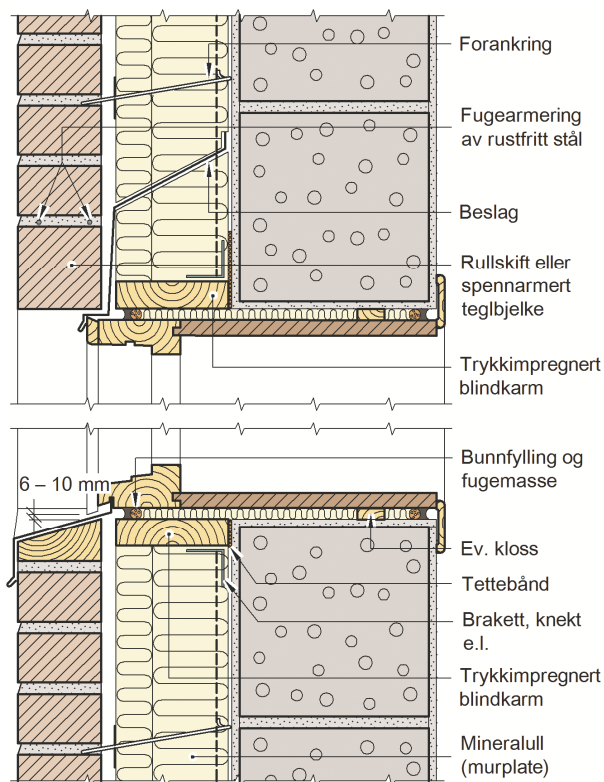
Fig. 441 Eksempel på tilslutning til vindu i murt vegg med utvendig etterisolering og murt forblending
