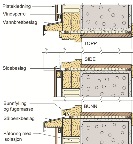
Fig. 361 a Eksempel på tilslutning til nytt vindu i murt vegg med utvendig påføring med isolasjon
