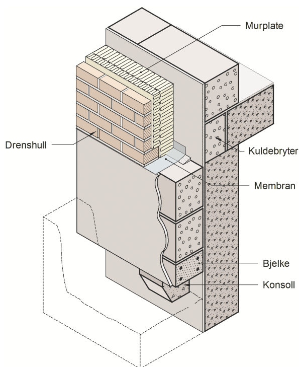
Fig. 442 Eksempel på opplegg for murt forblending med opplegg på plasstøp- te konsoller med betongbjelke mellom
