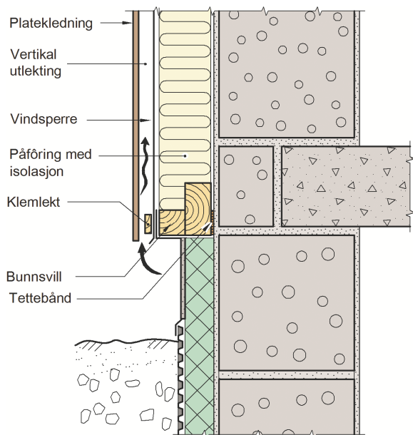
Fig. 363 Eksempel på tilslutning til fundament i murt vegg med utvendig påføring med isolasjon. Her er grunnmur/kjellervegg også etterisolert.
